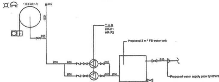
ELEVATION FOR AREA 'D' n.t.s.
