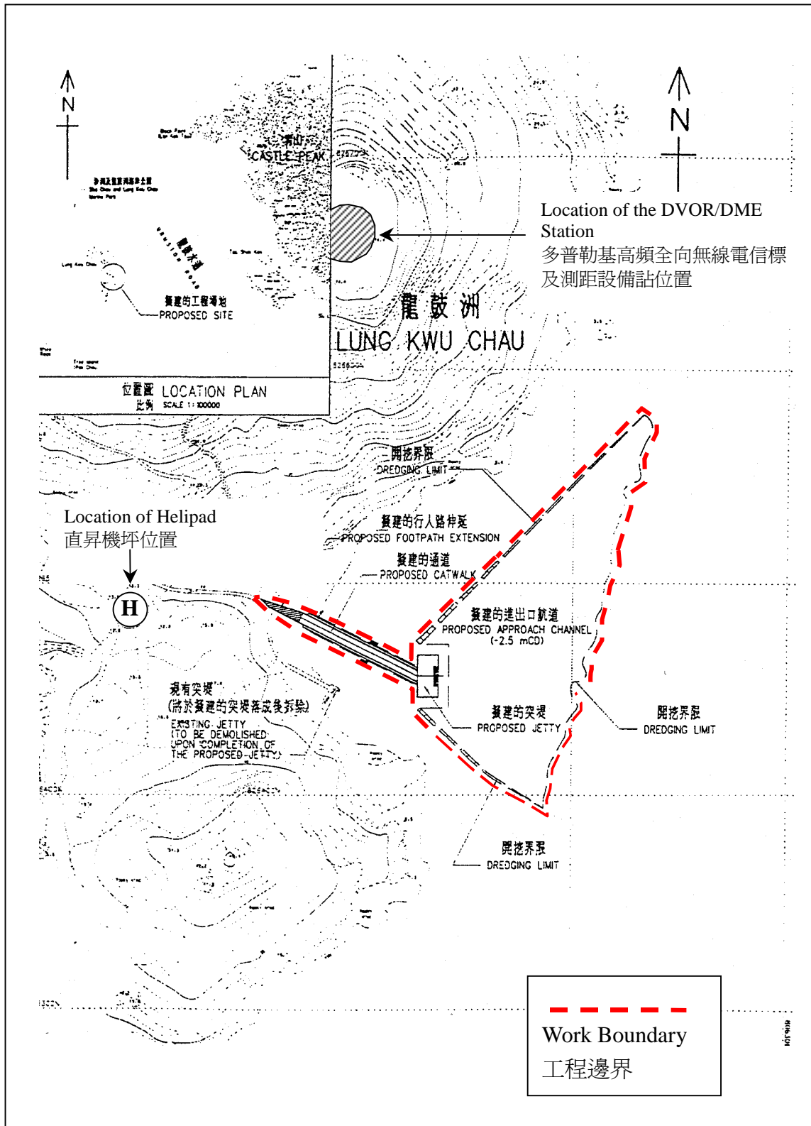
Figure 1 Construction of Lung Kwu Chau Jetty – Location Plan 圖 1 興建龍鼓洲突堤 — 位置圖
