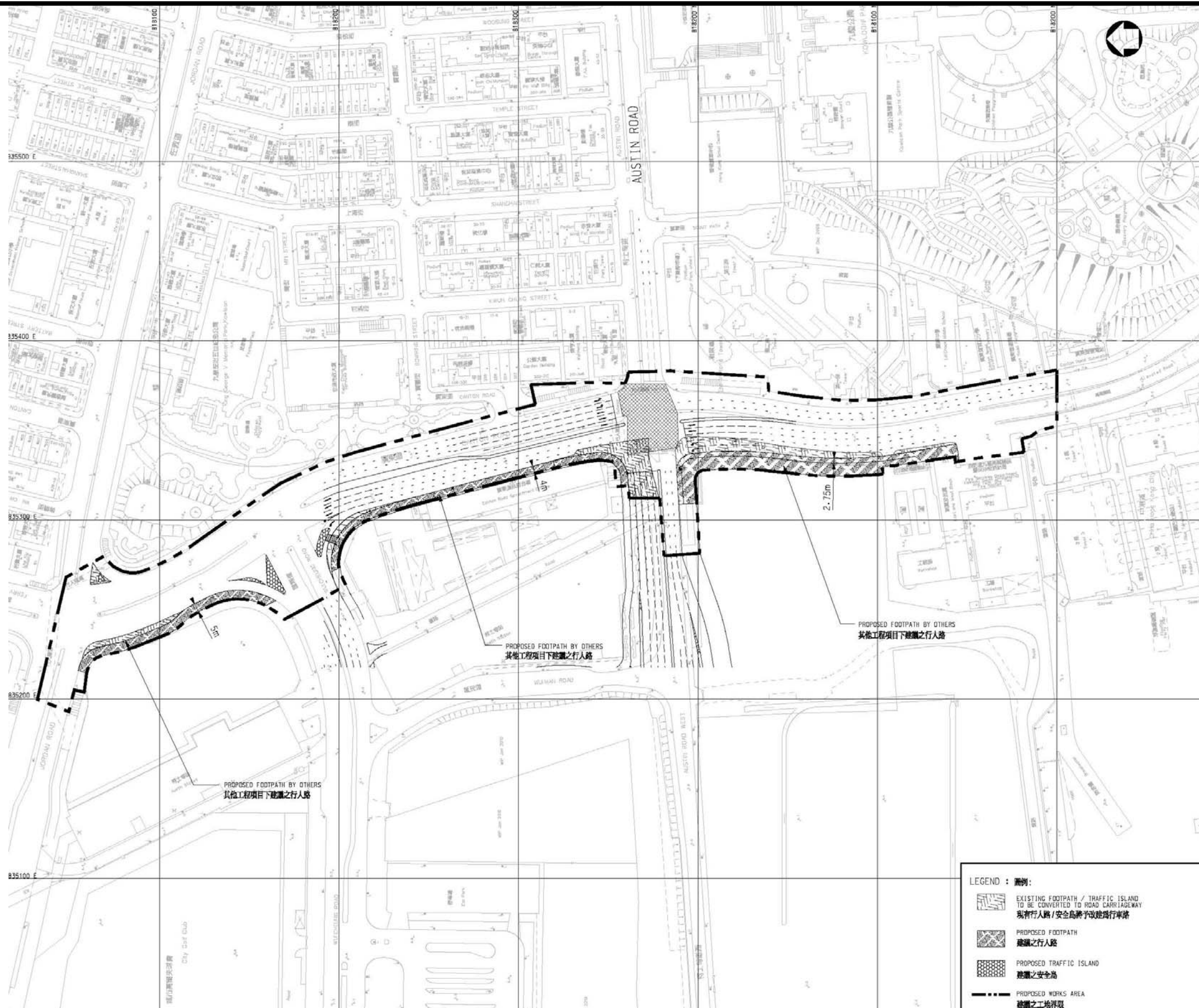
Figure 8: IMPROVEMENT WORKS AT CANTON ROAD - SCHEME Q INTERIM OPTION - ROAD LAYOUT PLAN 圖 八: 廣東道改善工程 - 計劃 Q 中期方案道路平面佈置圖
