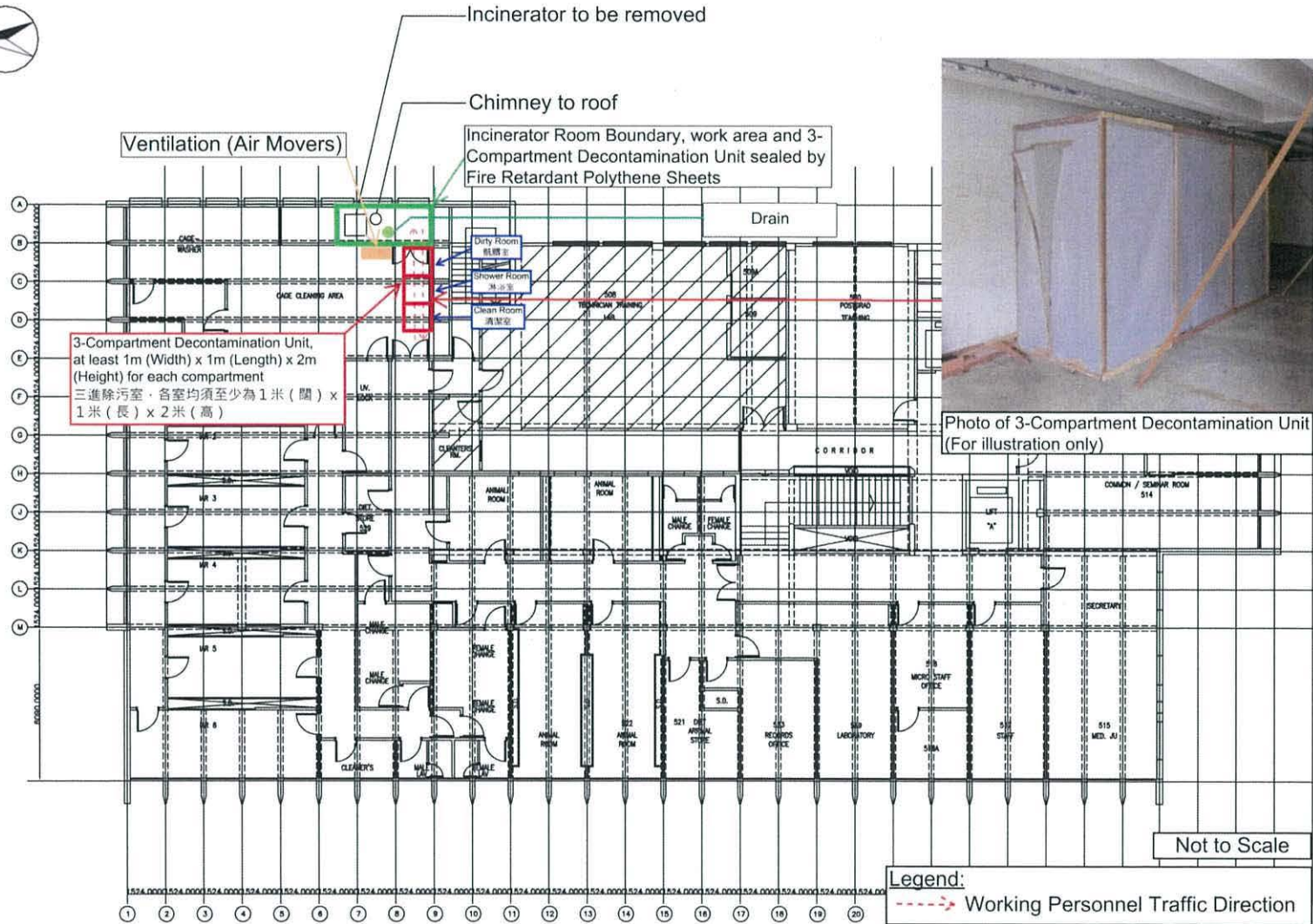
Figure 4: Floor Plan of the Incinerator Room in UPB 圖 4: 在大學病理學樓內的焚化爐房平面圖
