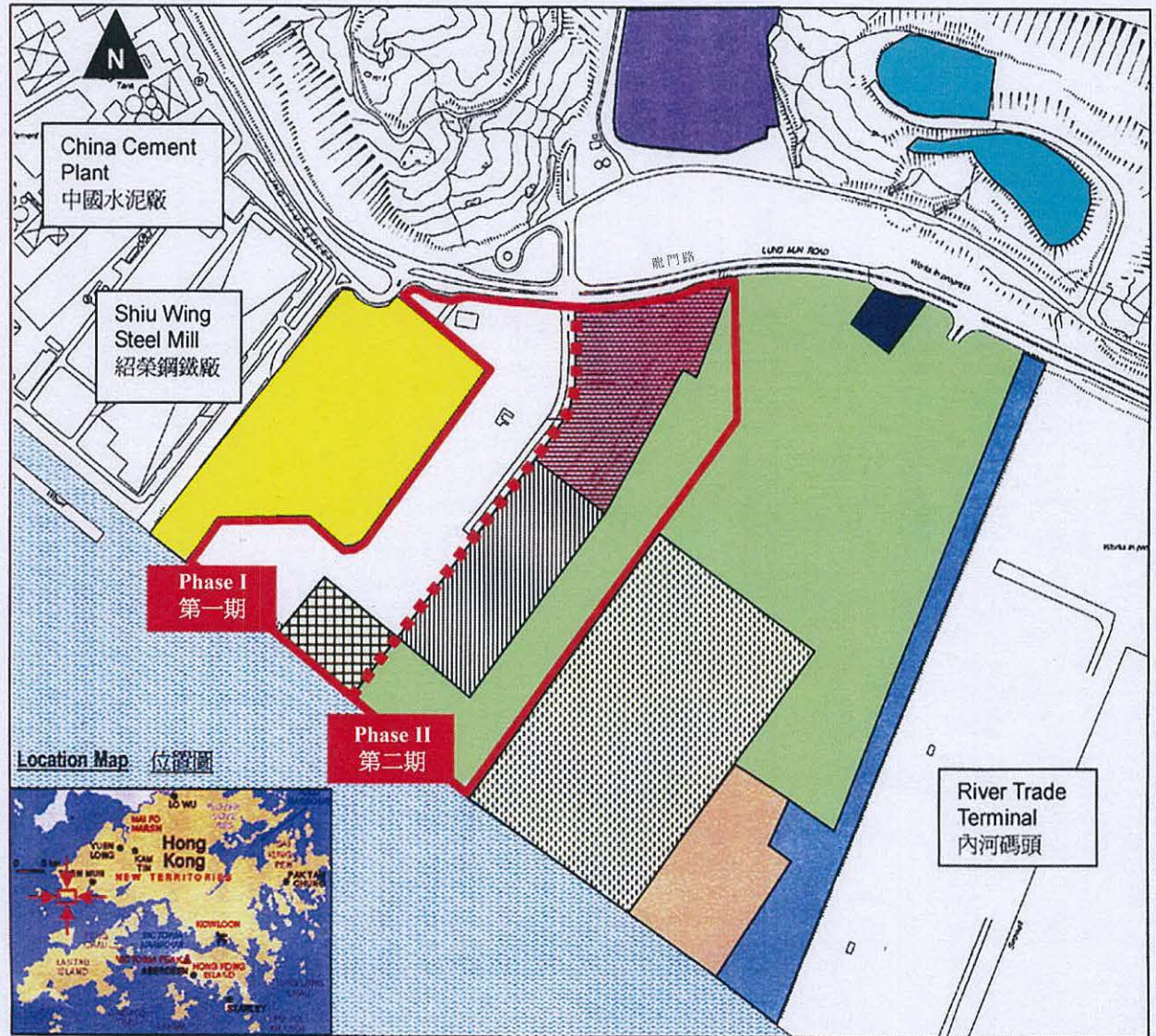
Development of an EcoPark in Tuen Mun Area 38 - Location of the EcoPark and Other Users 於屯門38區發展環保園 - 位於屯門38區的環保園及其他使用者位置圖
