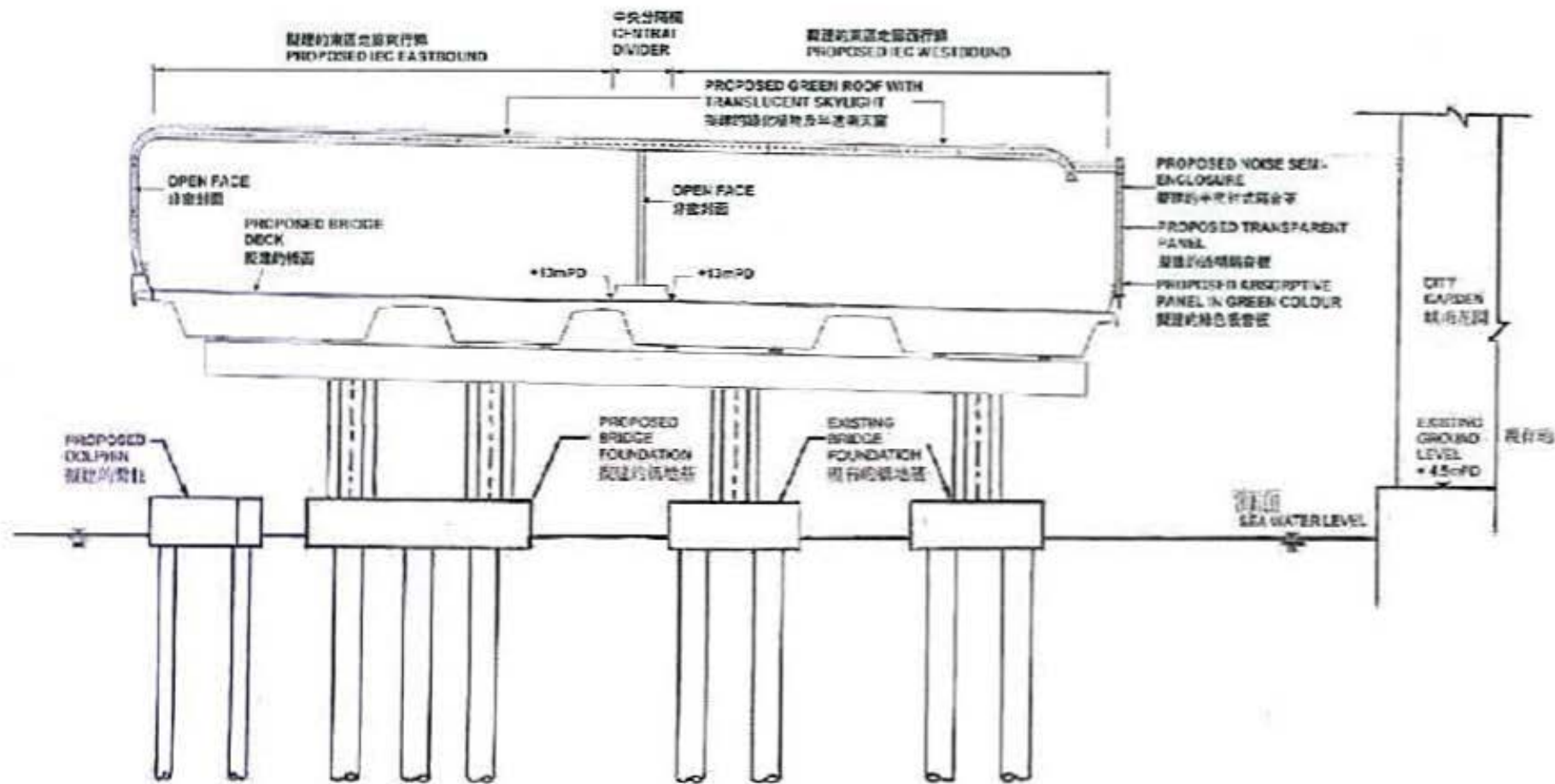
切面 C-C
