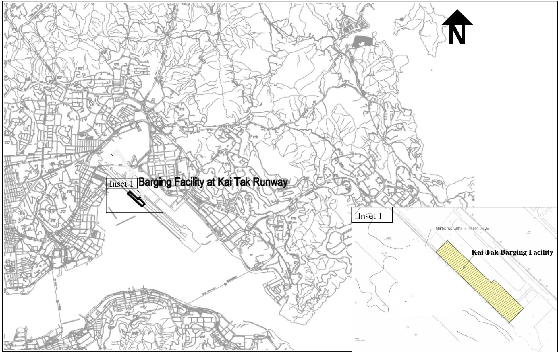
Figure 9b: Location of Works Areas (Off-Site) – Kai Tak Barging Facility 圖 9b: 工地外的工作區 – 啟德跑道躉船轉運站位置圖
