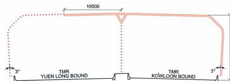
SECTION 11-11 SEMI-ENCLOSURE NM 18 (N.T.S.)
