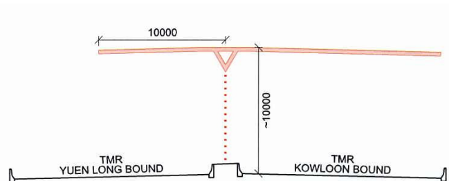
SECTION 10-10 SEMI-ENCLOSURE NM 17 (N.T.S.)
