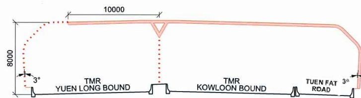
SECTION 9-9 SEMI-ENCLOSURE NM16 (N.T.S.)
