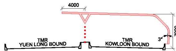
SECTION 6-6 SEMI-ENCLOSURE NM 11 (N.T.S.)
