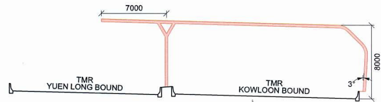
SECTION 2-2 FULL ENCLOSURE NM 2 (N.T.S.)
