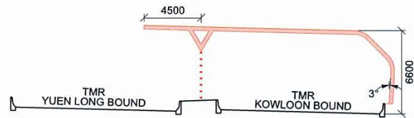
SECTION 1-1 SEMI-ENCLOSURE NM 1 (N.T.S.)
