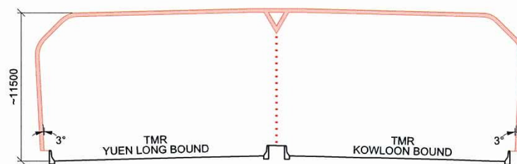
SECTION 15-15 FULL ENCLOSURE NM 24 (N.T.S.)
