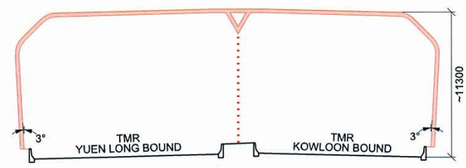
SECTION 12-12 FULL ENCLOSURE NM 19 (N.T.S.)
