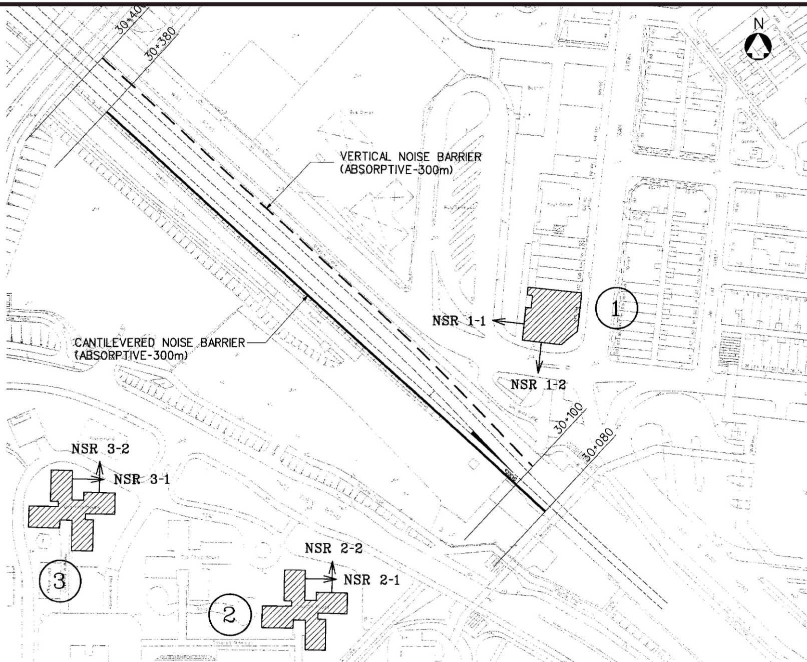
Figure 10 - Sheung Shui to Lok Ma Chau Spur Line (上水至落馬州支線) 圖十 - 條例3.27 所指之隔音屏障位置
