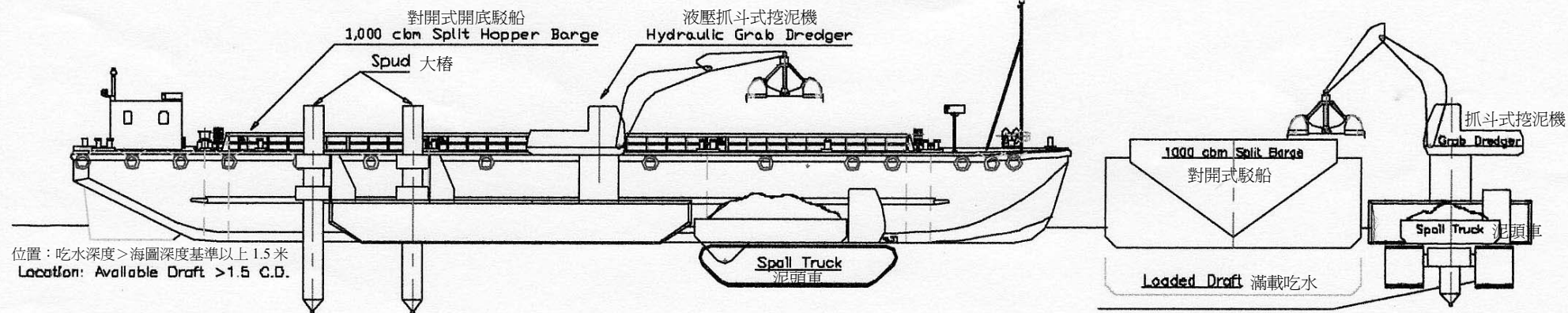
END VIEW-LOADING 端視圖 - 裝卸情況
