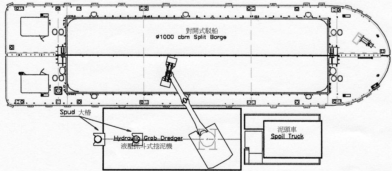
PLAN VIEW 俯視圖
