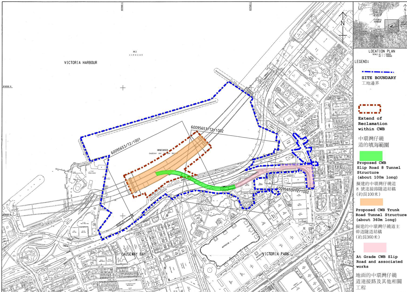
Figure 1b: General Layout of the Project 圖 1b : 工程項目佈局圖
