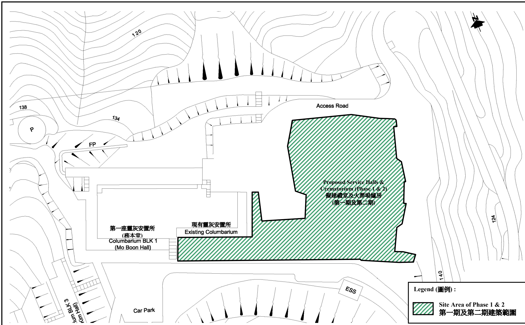
Figure 3: Block Plan of New Crematorium upon completion of Phase 1 & 2 圖 3: 在第一及第二期工程完成後新火葬場的平面圖
