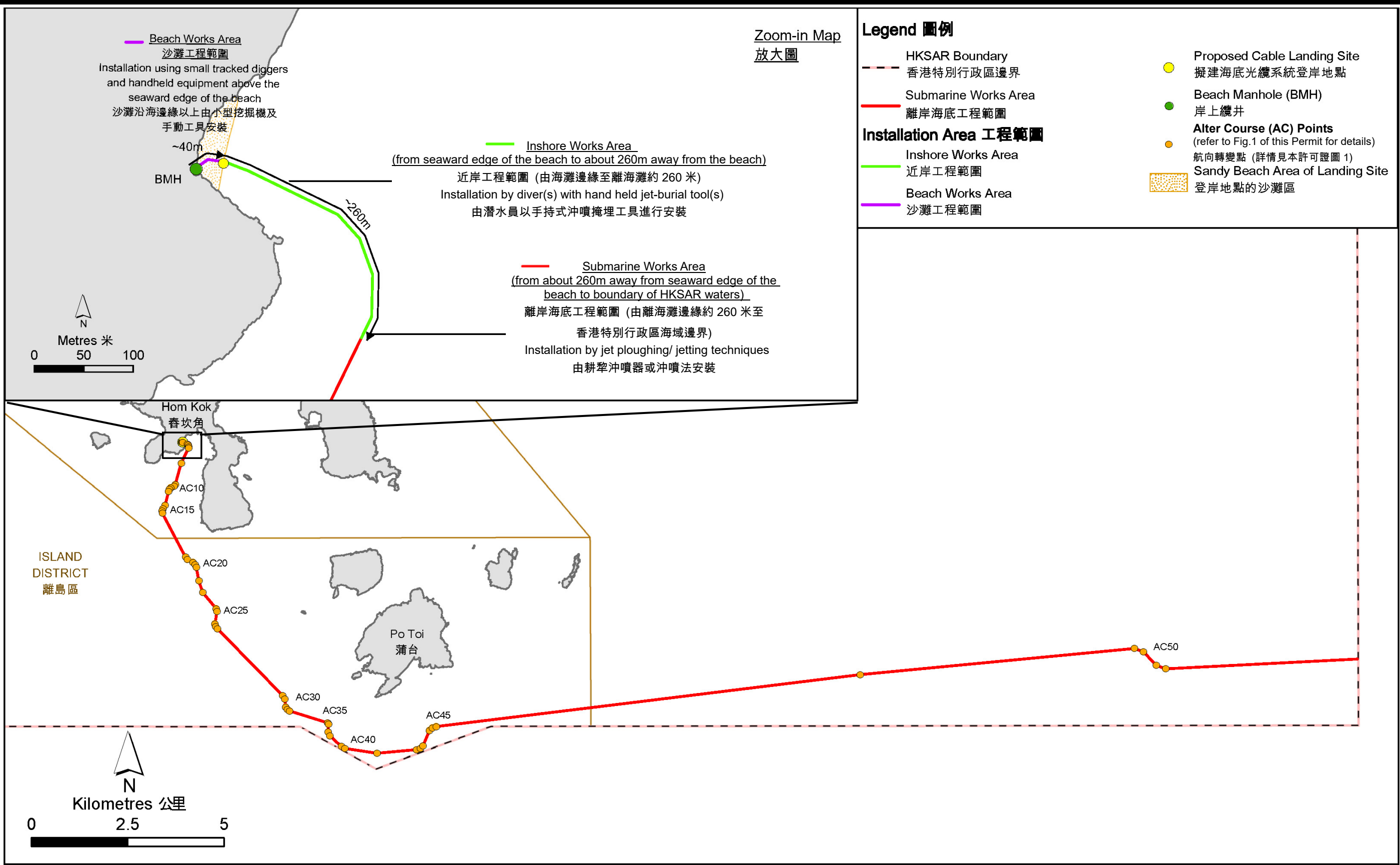
Project Title 工程項目名稱 H2H Express Submarine Cable 海南-香港光纜系統 Figure 3 圖 3 Installation Method of the Cable 光纜系統的安裝方法
