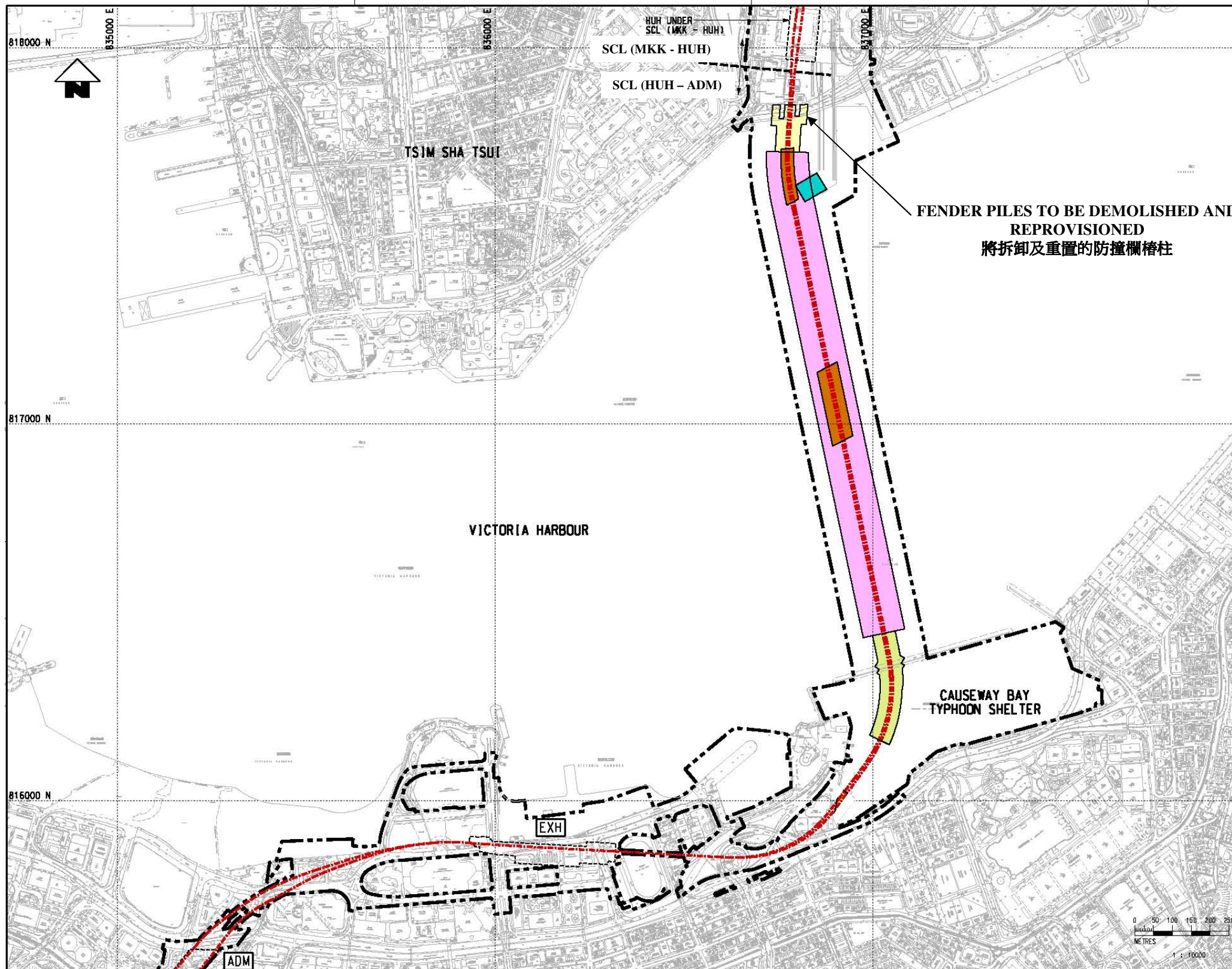
Figure 2: Marine Works for Shatin to Central Link – Hung Hom to Admiralty Section 圖 2: 沙田至中環綫 - 紅磡至金鐘段之海上工程
