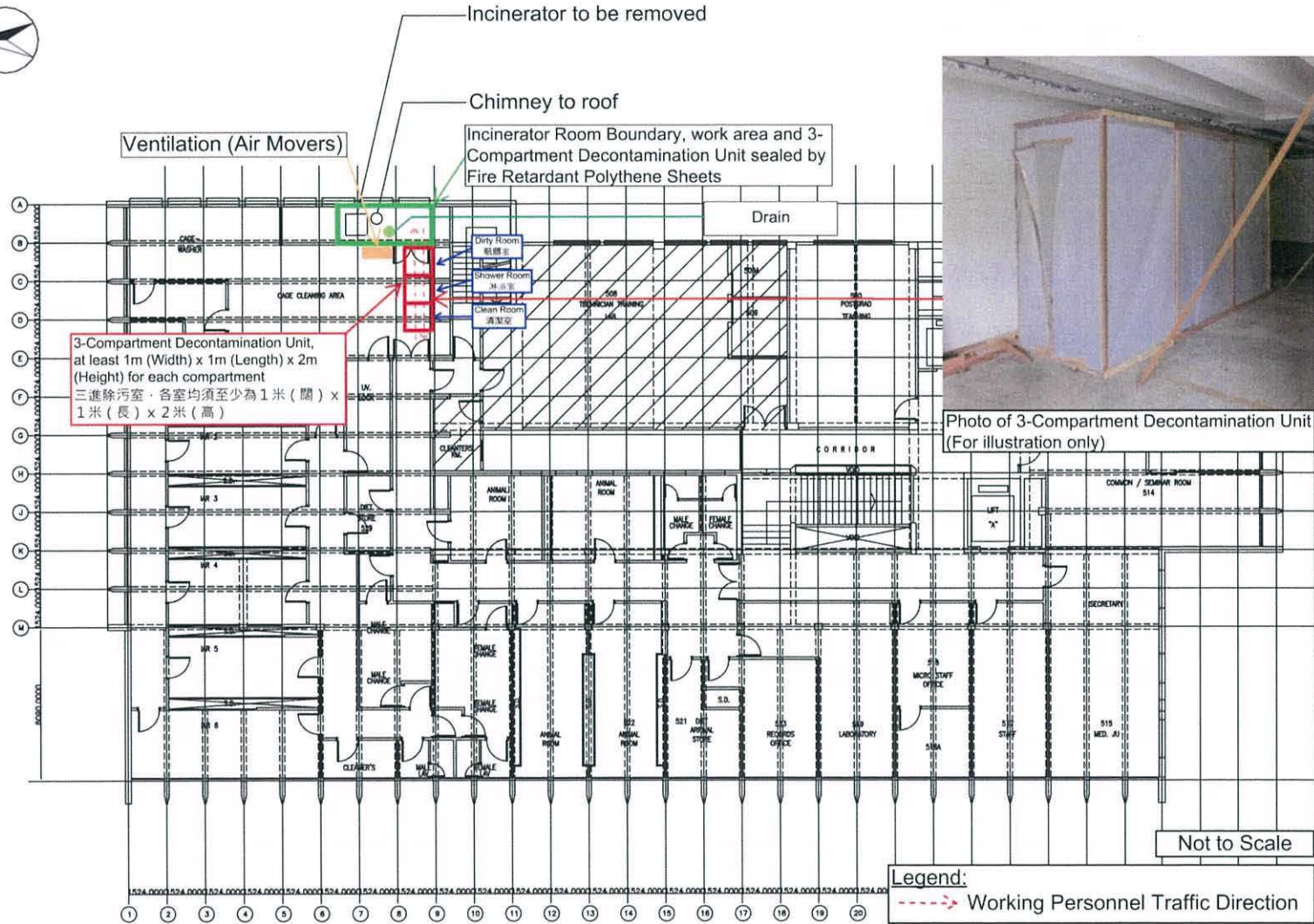
Figure 2: Floor Plan of the Incinerator Room in UPB 圖 2: 在大學病理學樓內的焚化爐房平面圖
