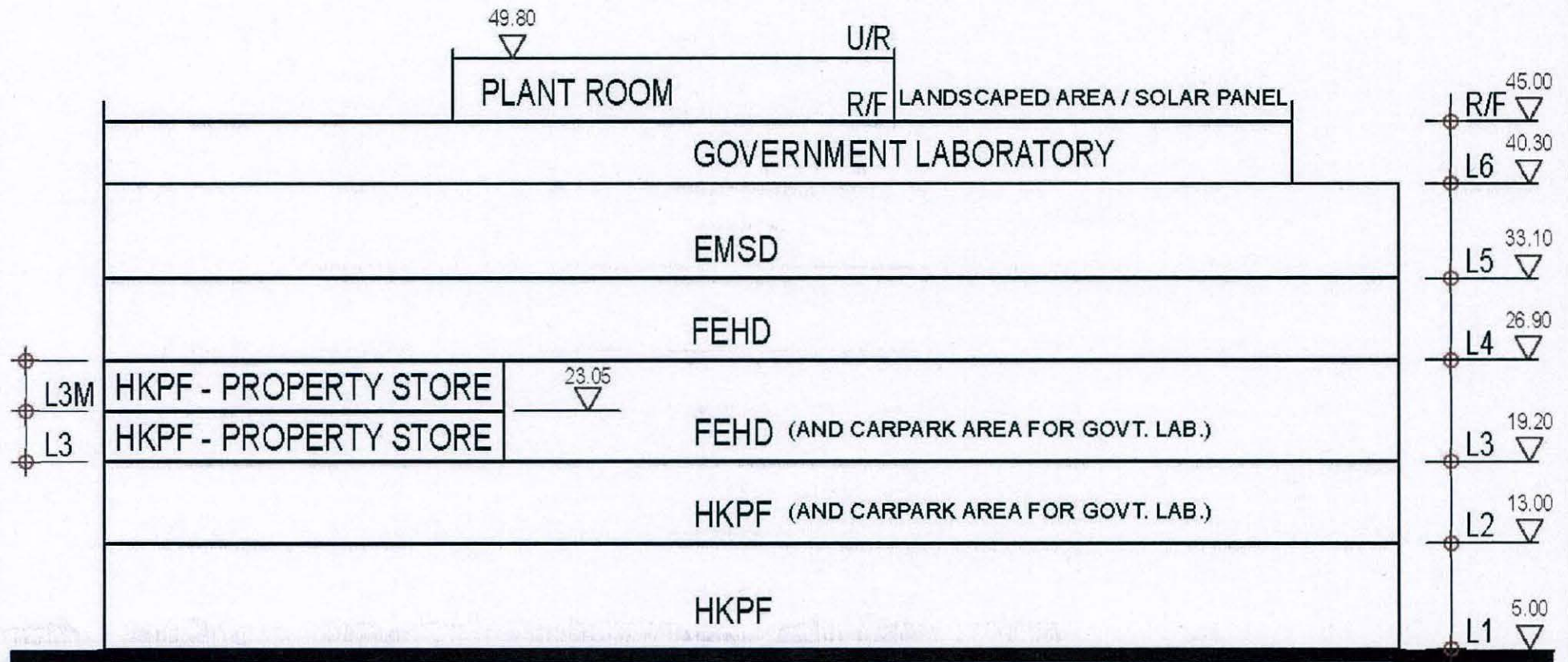
Typical Section A-A N.T.S
