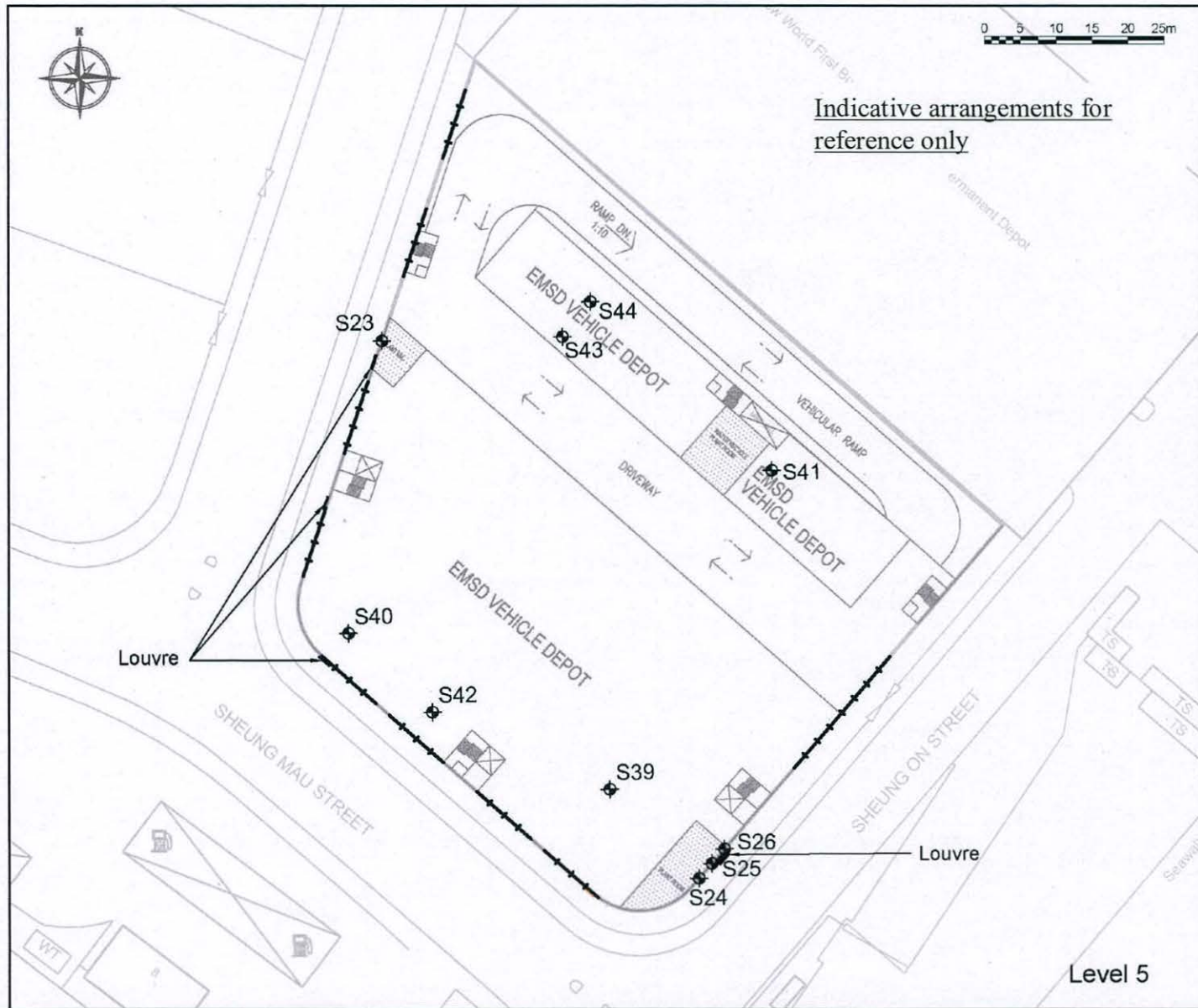
Figure 3: General Layout Plan of EMSD vehicle depot. 圖 3: 機電工程署修理車廠佈局圖
